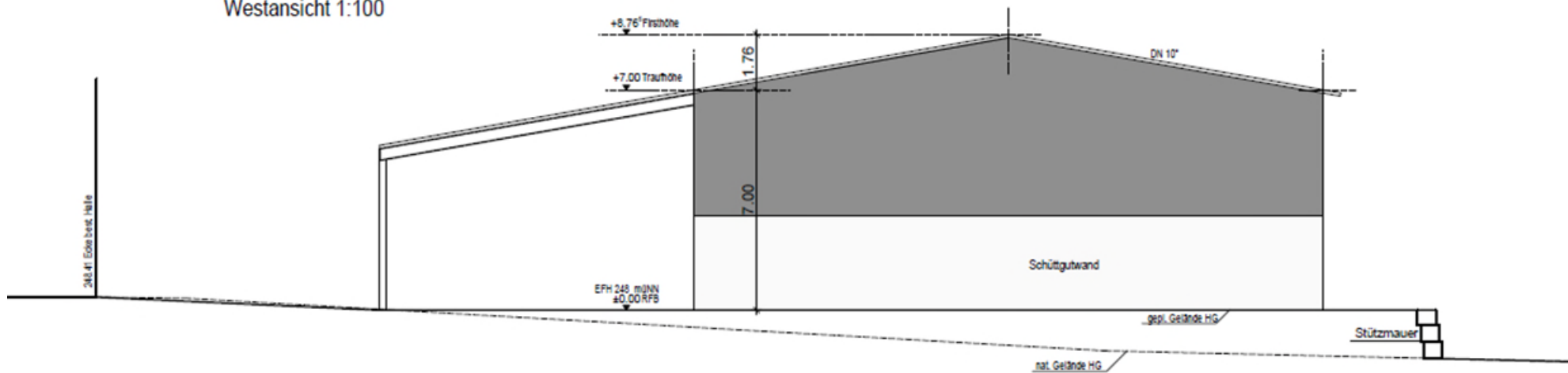
Ansicht West
