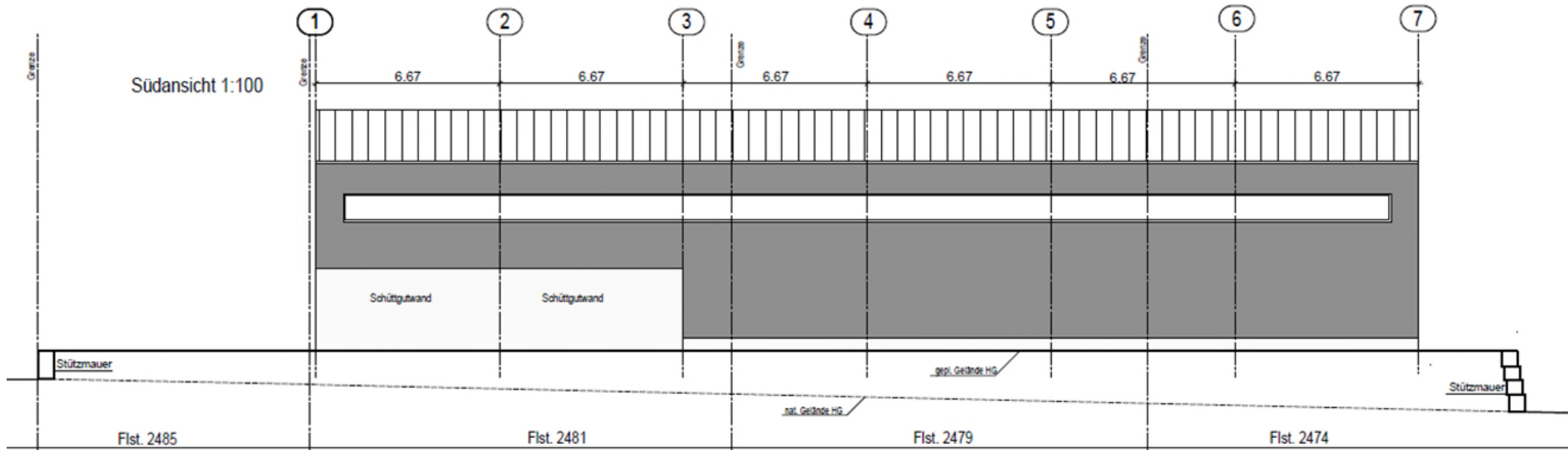
Ansicht Süd
